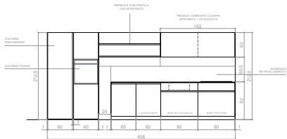
VISTA FRONTALE LATI COLONNE
