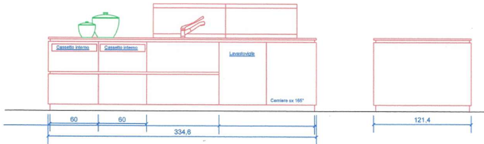
Prospetto F
