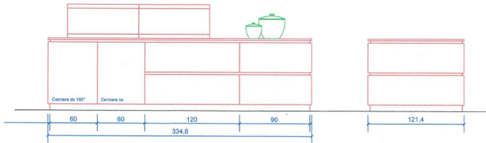
Prospetto D
