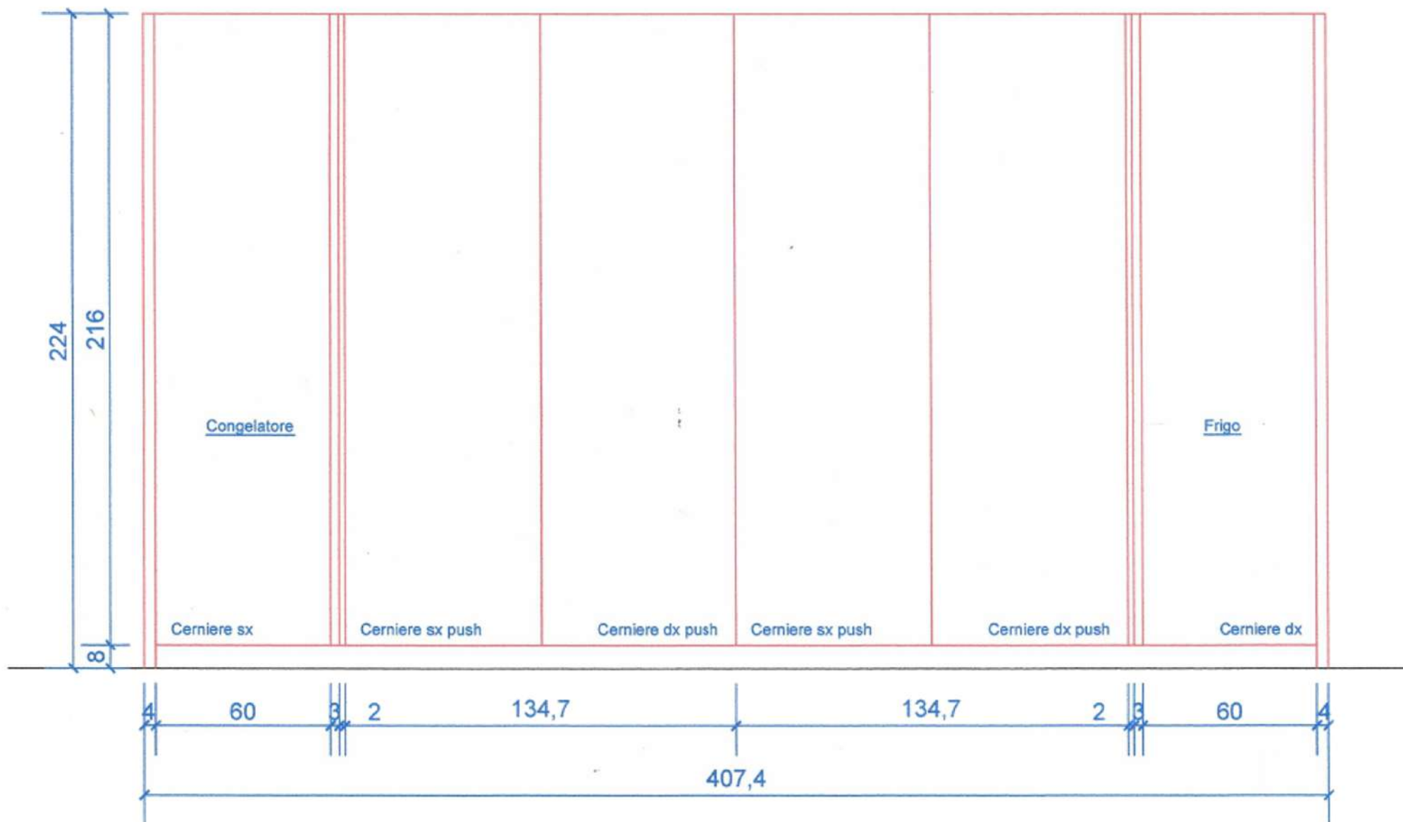
Prospetto C
