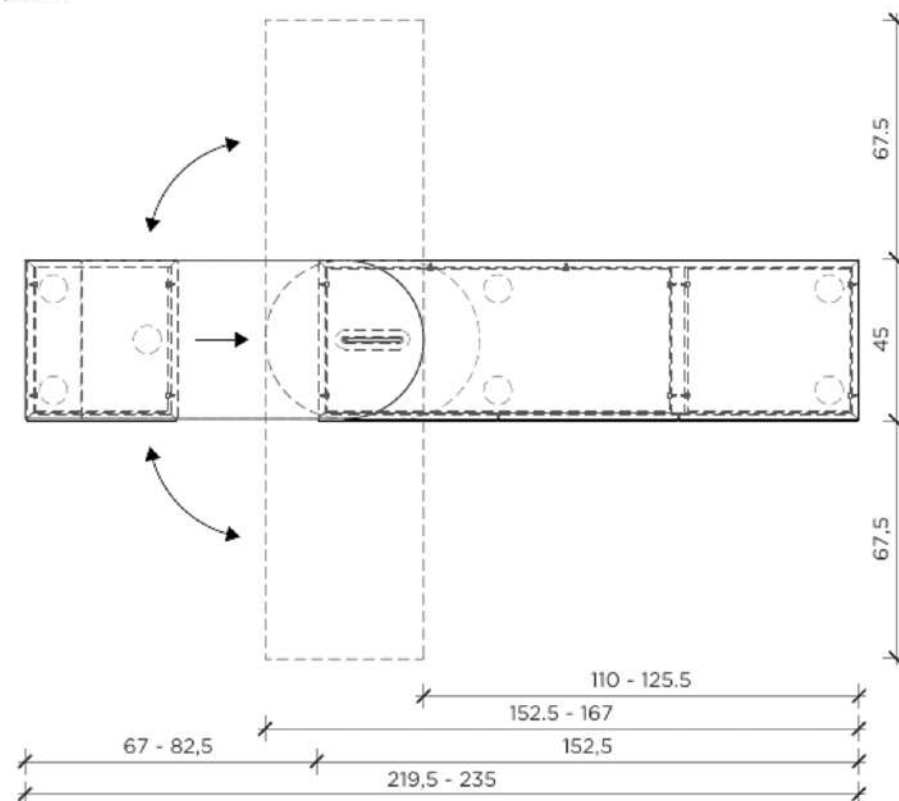
PIANTA | PLAN
