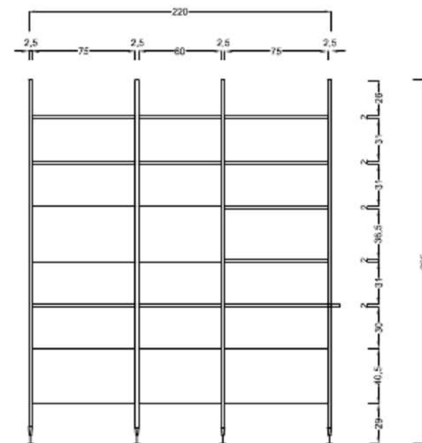
PROSPETTO F
