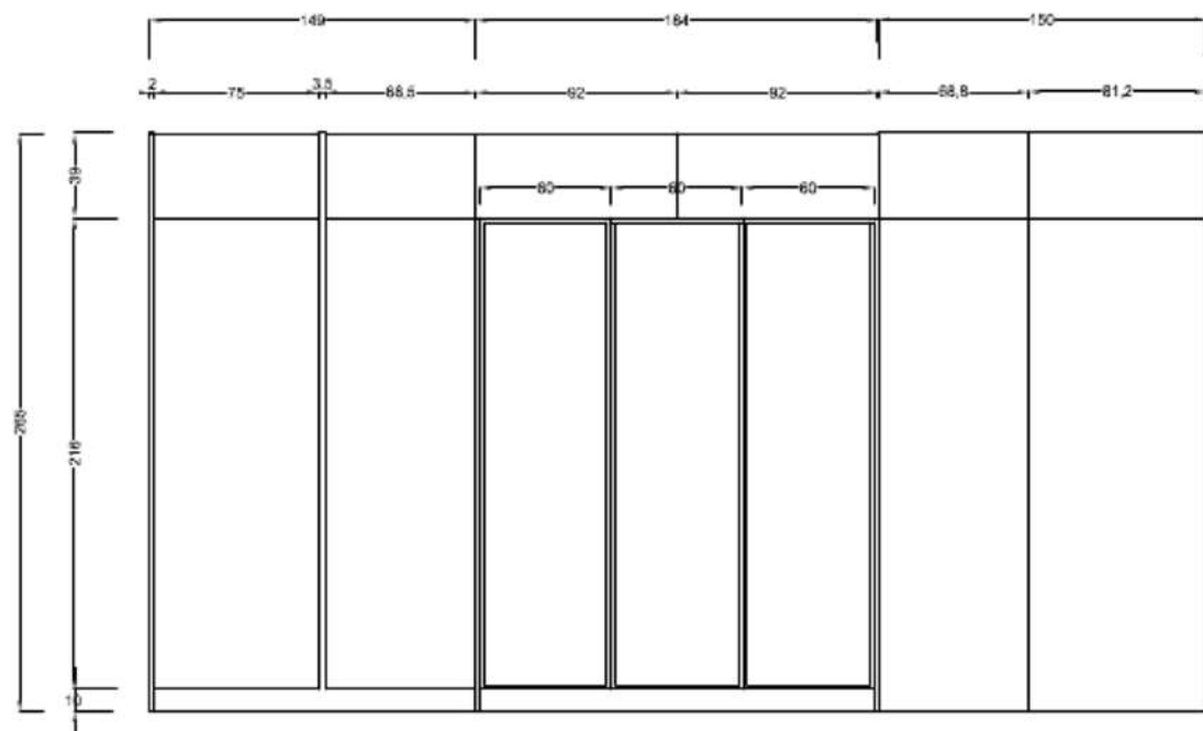
PROSPETTO E
