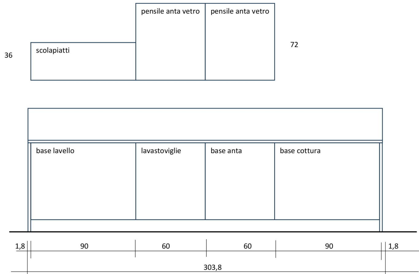
vista frontale
