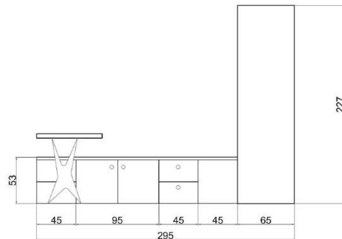
SEZ. A-A
