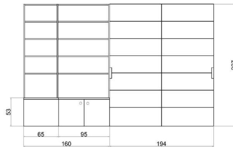
SEZ. B-B
